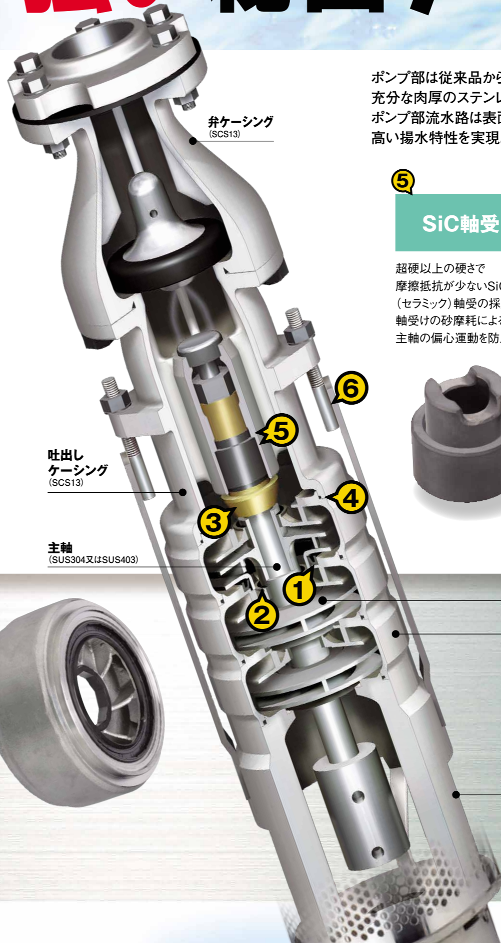
インペラ (SCS13)
