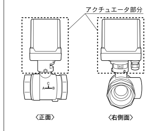
MAC3-130A ボール弁
