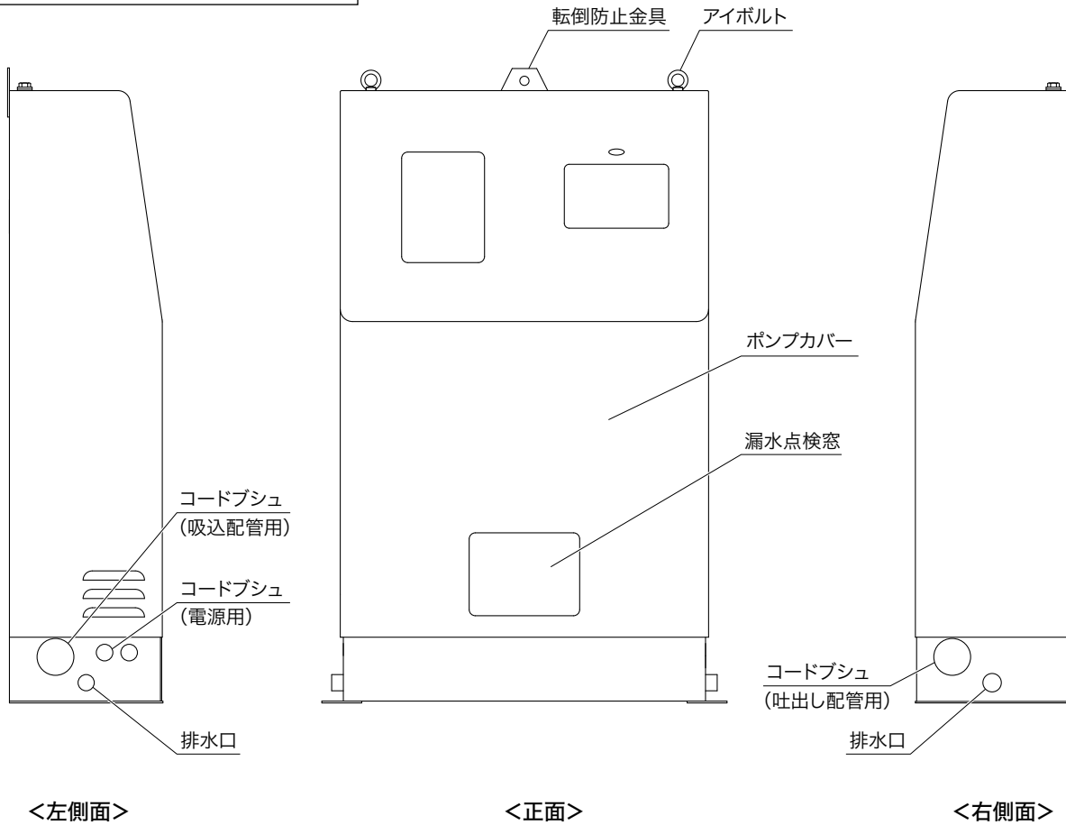
製品全体図【NDP2-G形 標準品】
