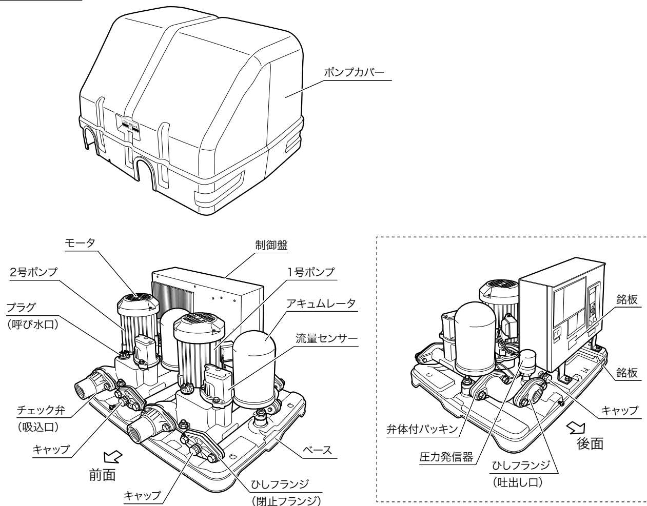
製品全体図
