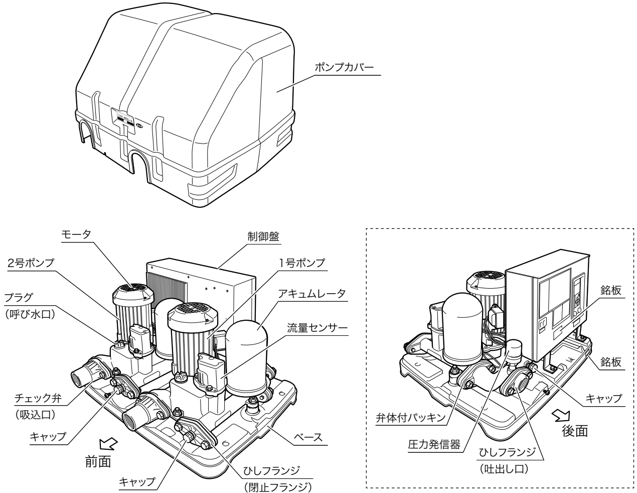
製品全体図
